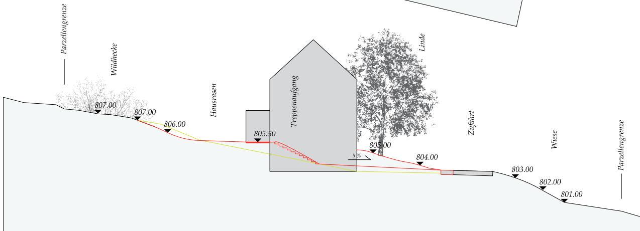
Schnitt A-A' Mst. 1:250
