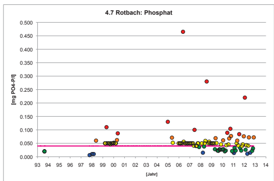
Fig. 56: Verlauf der Phosphatkonzentration im Zeitraum 1993-2013 an der Stelle 4.7 am Rotbach im Gmündentobel.
