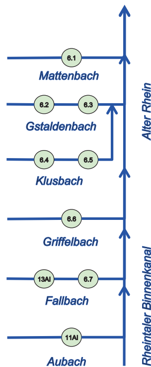
Fig. 80: Gewässersystem, Probenahmestellen, (ARA's gibt es keine) im Einzugsgebiet der appenzellischen Zuflüsse des Alten Rheins und des Rheintaler Binnenkanals.
