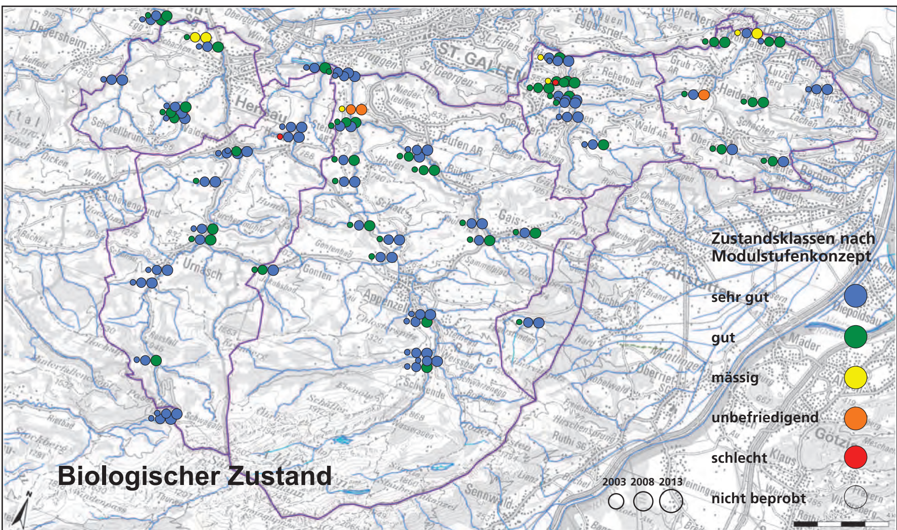
Abb. 2: Zustand der appenzellischen Gewässer 2013 im biologischen Aspekt (Makrozoobenthos und Kieselalgen), bezogen auf die ökologischen Ziele der GSchV (Anhang 1): Bewertet wurde immer der schlechteste Parameter nach der fünfstufigen Skala. Gezeigt werden auch die Veränderungen seit 2003 (kleine [2003], mittlere [2008] und grosse [2013] Kreise).
