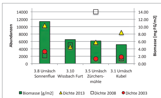
Fig. 29: Biomasse 2013 und Gesamtindividuendichte 2002-2013 des Makrozoobenthos an den 3 Stellen der Urnäsch und am Wissbach.
