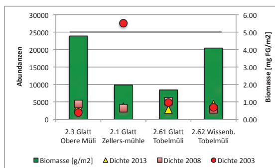
Fig. 15: Biomasse 2013 und Gesamtindividuendichte 2003-2013 des Makrozoobenthos an den 3 Stellen der Glatt und am Wissenbach.
