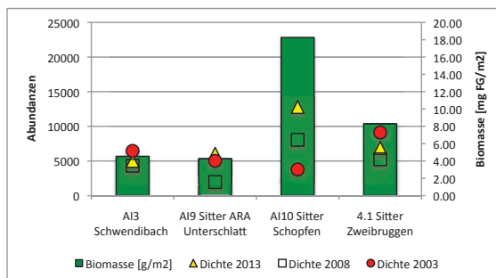
Fig. 45: Biomasse 2013 und Gesamtindividuedichte 2003-2013 des Makrozoobenthos an den 4 Stellen der Sitter.
