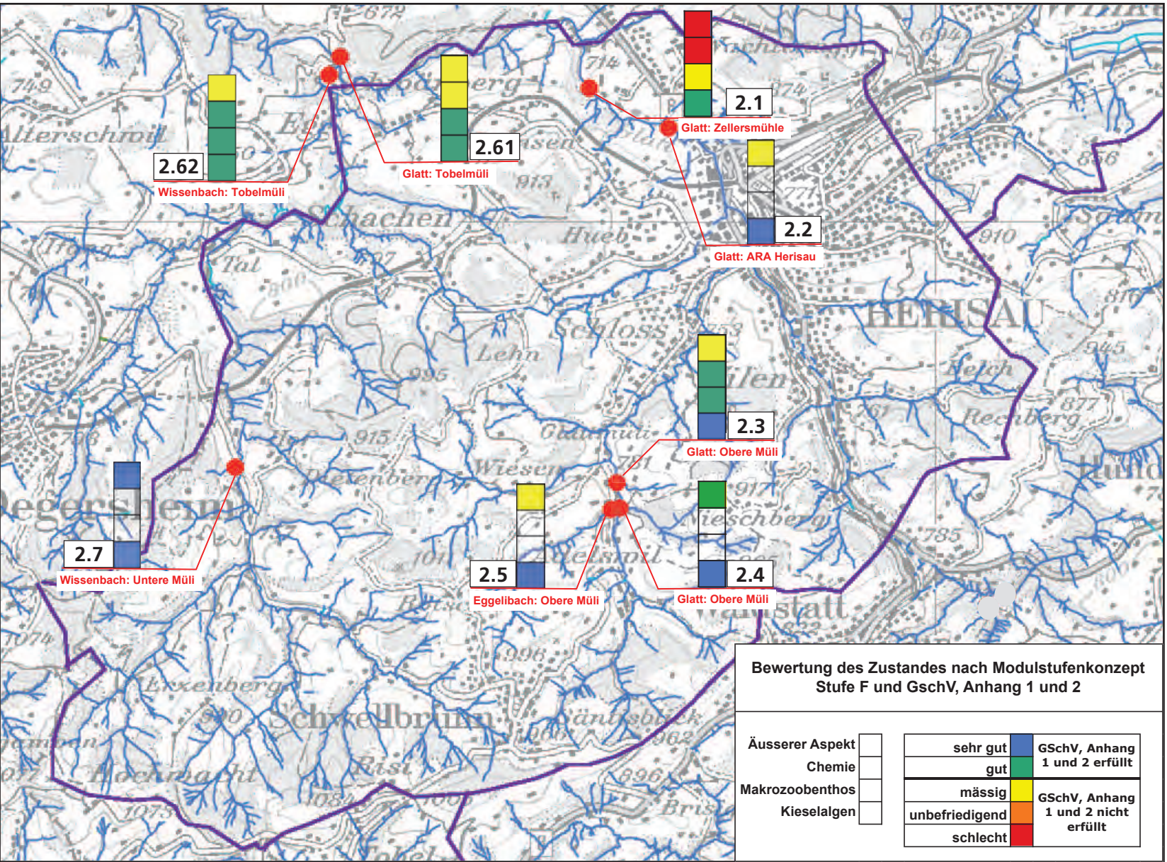
Abb. 4: Zustand der Gewässer an den Probennahmestellen im Einzugsgebiet der Glatt gemäß dem Äusserem Aspekt, der Chemie (Anhang 2 GSchV), dem Makrozoobenthos und der Kieselalgen. Ausschlaggebend für die Bewertung war immer der schlechteste Parameter.
