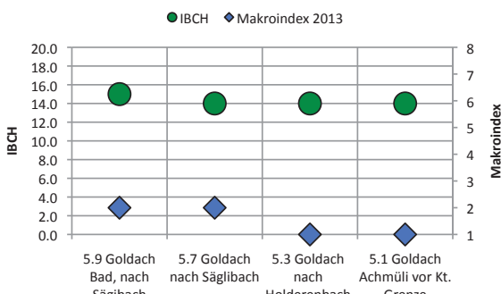
Fig. 74: IBCH und Makroindex 2013 an den 4 Stellen im Einzugsgebiet der Goldach.
