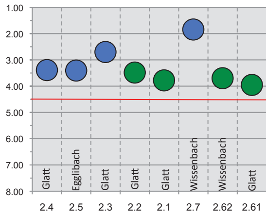
Fig. 17: Biologische wirksame Belastung der Gewässer nach DI-CH im Einzugsgebiet der Glatt 2013. Das ökologische Ziel der GSchV ist erfüllt, wenn der DI-CH kleiner als 4.5 ist (rote Linie). Dies ist bei allen blauen und grünen Kreisen zutreffend.
