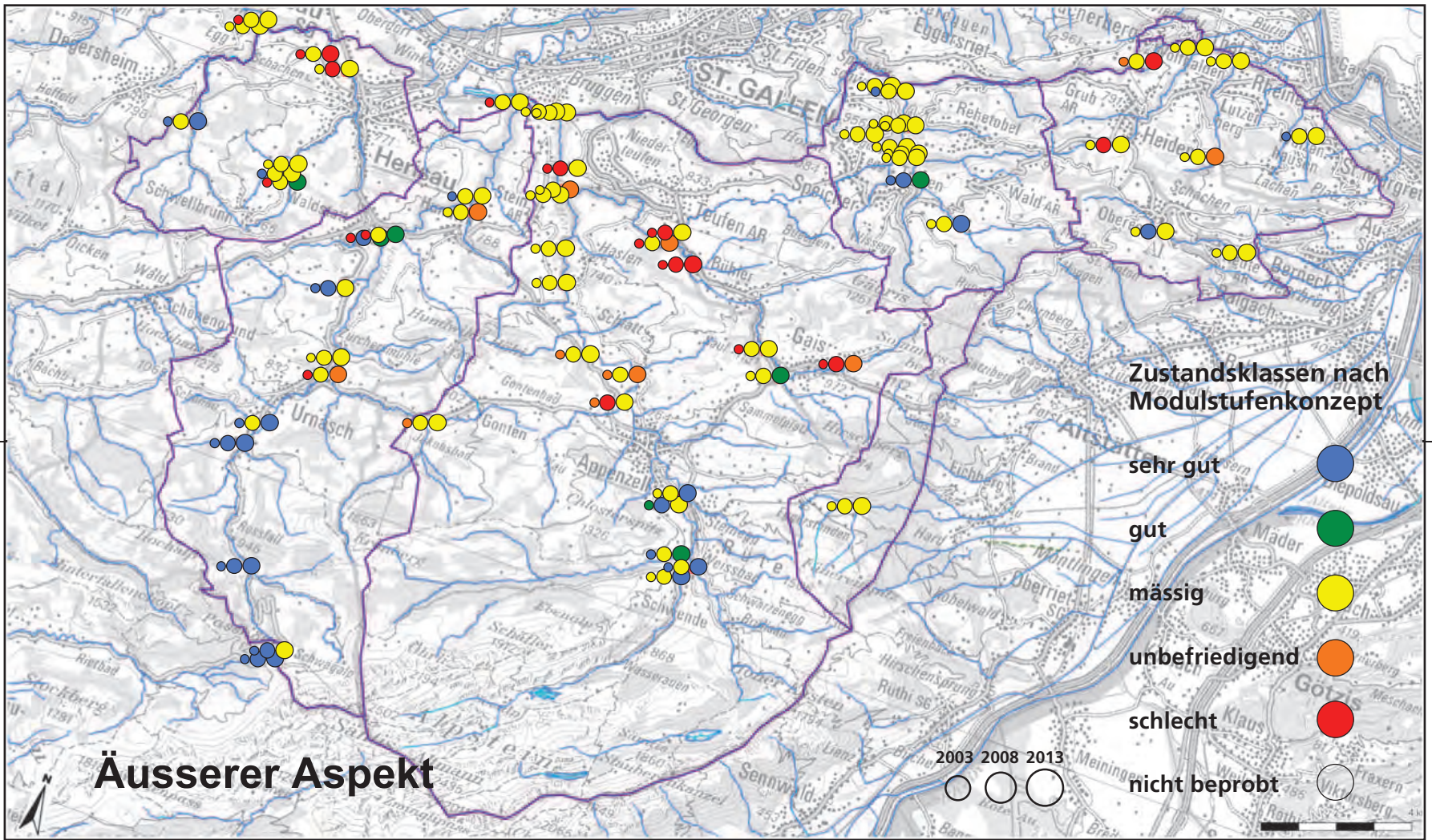
Abb. 1: Zustand 2013 der appenzellischen Gewässer im Äusseren Aspekt, bezogen auf die Anforderungen der GSchV (Anhang 2): Bewertet wurde immer der schlechteste Parameter. Der heterotrophe Bewuchs wurde nach der fünfstufigen, alle andern Parameter nach der dreistufigen Skala bewertet. Wo der heterotrophe Bewuchs ausschlaggebend war wurde auch die fünfstufige Skala verwendet. Gezeigt werden auch die Veränderungen seit 2003 (kleine [2003], mittlere [2008] und grosse [2013] Kreise).
