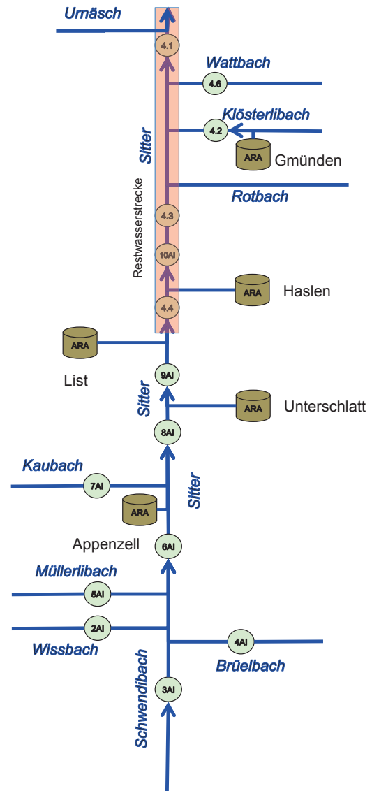
Fig. 33: Gewässersystem, Probenahmestellen und ARA-Einleitungen im Einzugsgebiet des Sitter (ohne EZG Rotbach).
