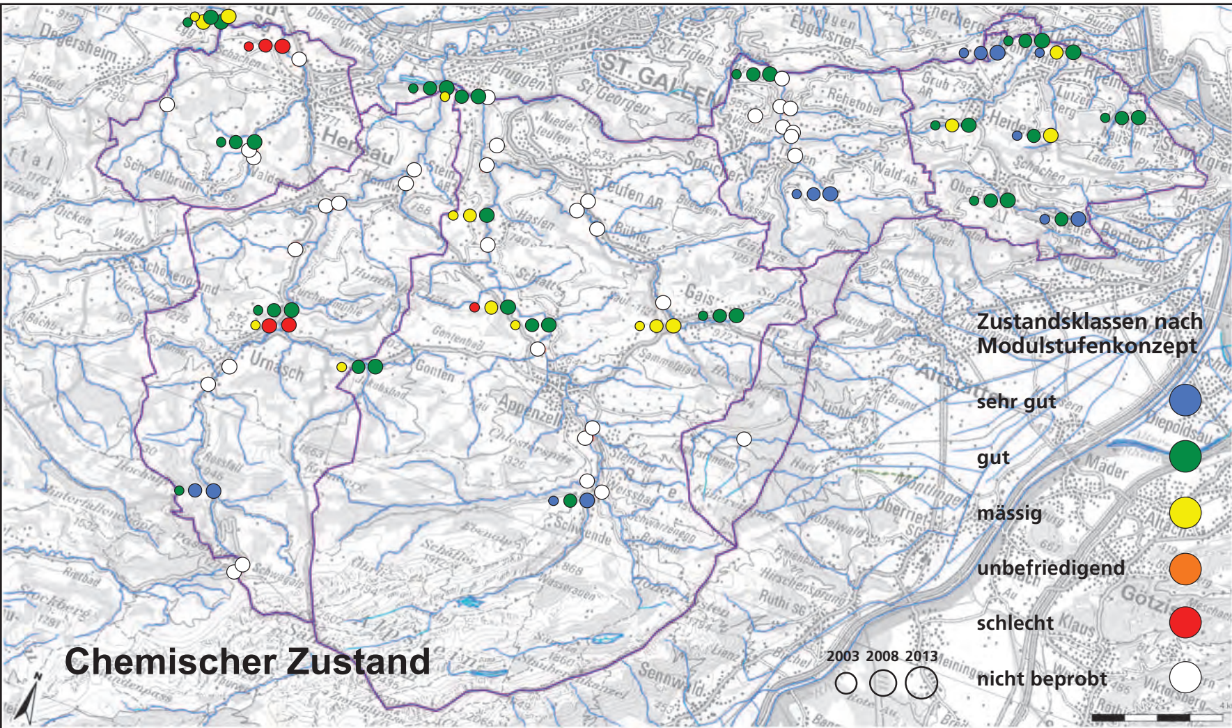
Abb. 3: Chemischer Zustand der appenzellischen Gewässer 2013, bezogen auf die Anforderungen (Anhang 2) der GSchV: Bewertet wurde immer der schlechteste Parameter nach der fünfstufigen Skala. Gezeigt werden auch die Veränderungen seit 2003 (kleine [2003], mittlere [2008] und grosse [2013] Kreise).
