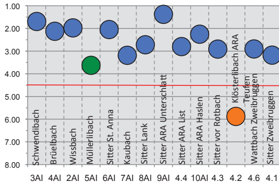
Fig. 47: Gesamtbelastung der Gewässer nach DI-CH im Einzugsgebiet der Sitter 2013. Das ökologische Ziel der GSchV ist erreicht, wenn der DI-CH kleiner als 4.5 ist. Dies ist bei allen blauen und grünen Kreisen der Fall.
