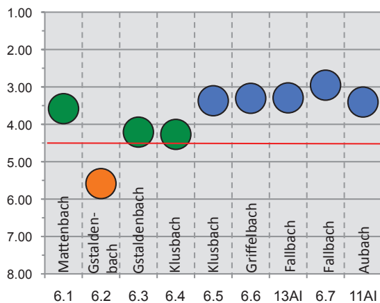
Fig. 91: Gesamtbelastung der Gewässer im Einzugsgebiet des Rheintaler Binnenkanals 2013. Das ökologische Ziel der GSchV ist erfüllt, wenn der DI-CH kleiner als 4.5 ist. Dies ist bei allen blauen und grünen Kreisen der Fall.
