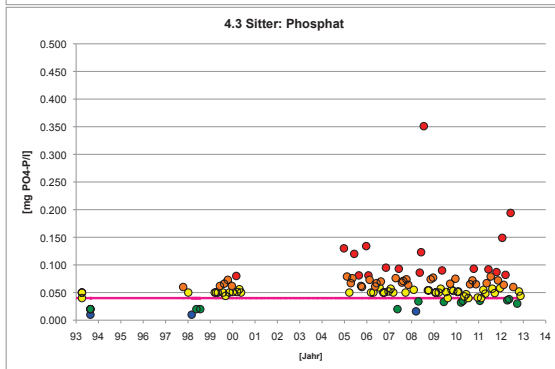
Fig. 40: Verlauf der Phosphatkonzentration im Zeitraum 1993-2013 an den Stellen Sitter 4.3 und 4.1.
