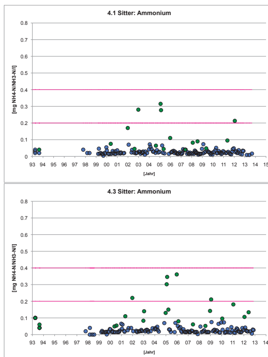
Fig. 36: Verlauf der Ammoniumkonzentration im Zeitraum 1993-2013 an den Stellen der Sitter vor dem Zufluss des Rotbaches (4.3) und nach dem Zufluss des Wattbaches (4.1)
