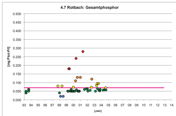
Fig. 55: Verlauf der Gesamtphosphor-Konzentration im Zeitraum 1993-2005 an der Stelle 4.7 am Rotbach im Gmündentobel.
