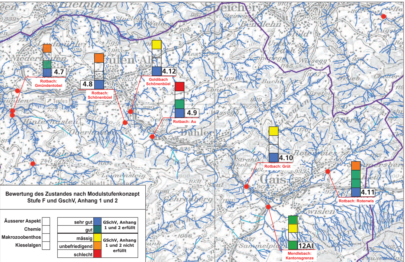
Abb. 7: Zustand der Gewässer an den Probenahmestellen im Einzugsgebiet des Rotbaches gemäß dem Äusseren Aspekt, der Chemie (Anhang 2 GSchV), dem Makrozoobenthos und der Kieselalgen. Ausschlaggebend für die Bewertung war immer der schlechteste Parameter.
