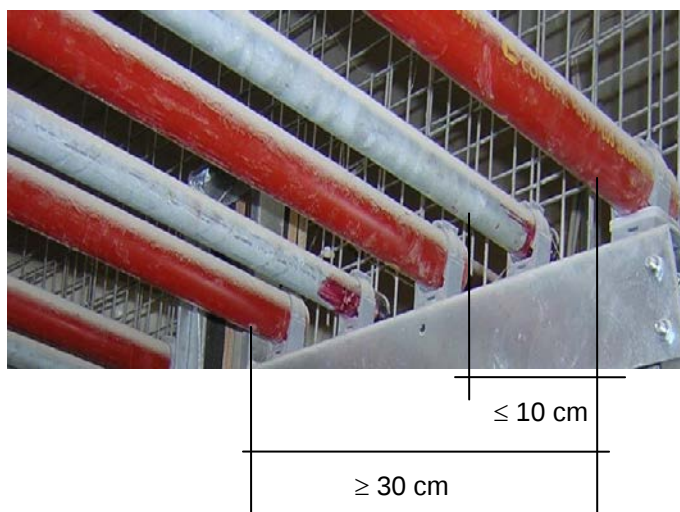
Abb. 5a Lattenrost aus Metallrohren
